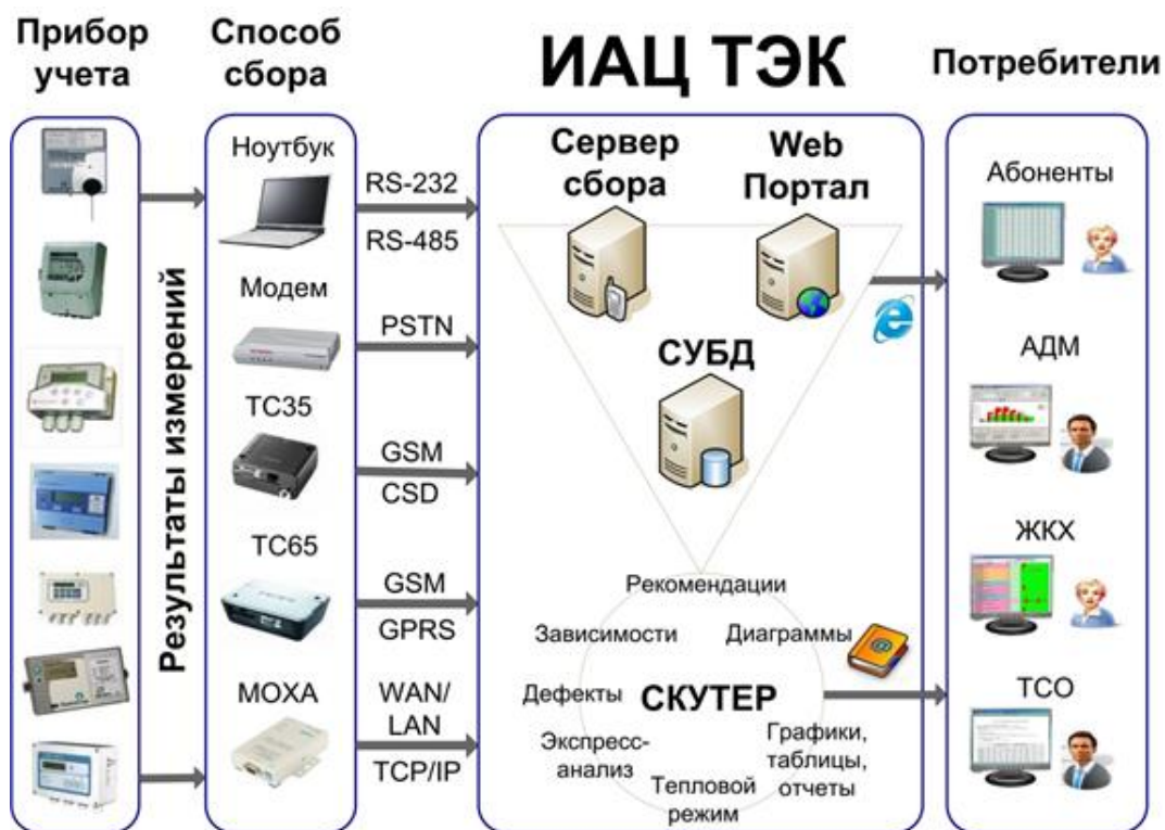
Рисунок 1. Структура системы диспетчеризации
